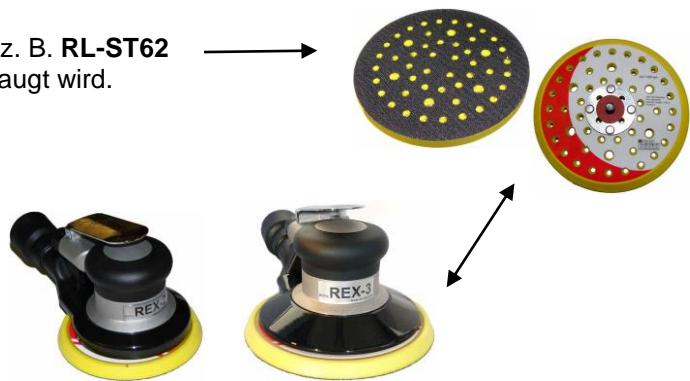
REX-2 (Ø 125 mm) REX-3 (Ø 150 mm) mit großer Absaugglocke
